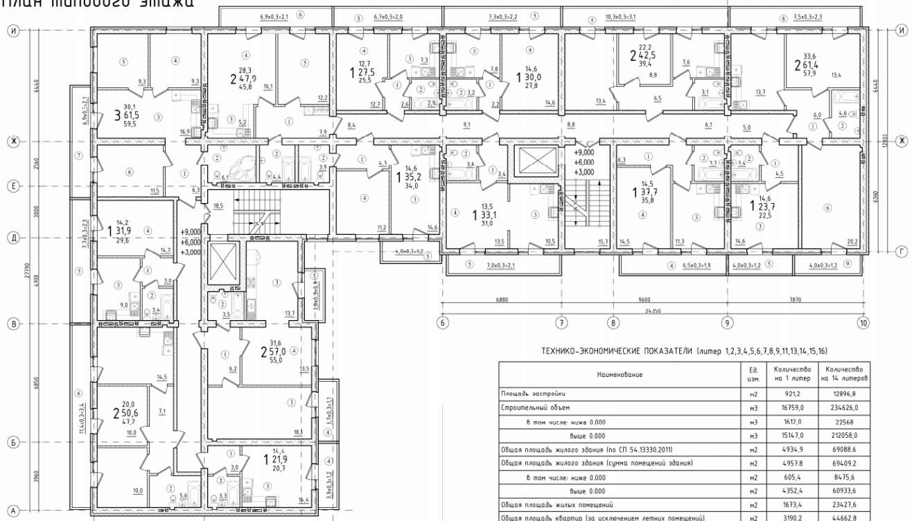
План типового этажа
